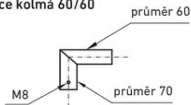
Redukce kolmá 60/60
