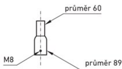
Redukce přímá 76/48
